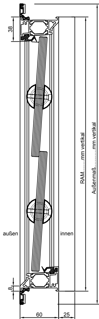
Vertikalschnitt
