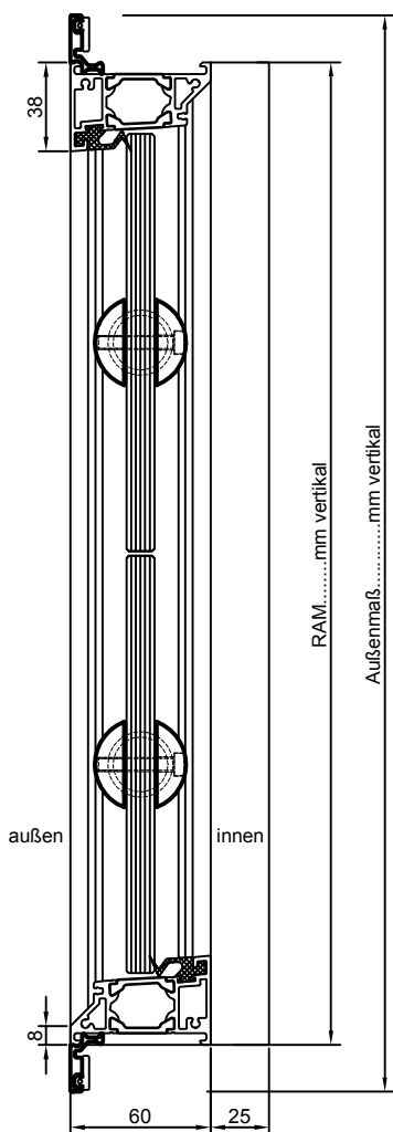
Vertikalschnitt
