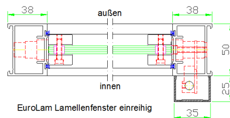
Horizontalschnitt
