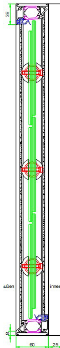
Vertikalschnitt
