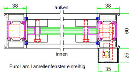
Horizontalschnitt
