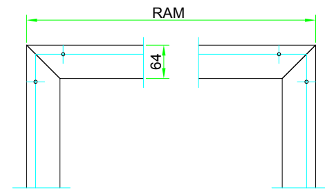
Ansicht Zarge
