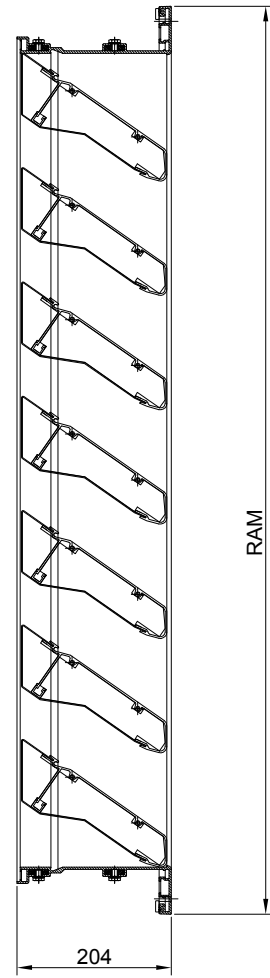
Vertikalschnitt
