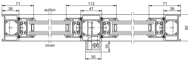
EuroLam Lamellenfenster zweireihig
