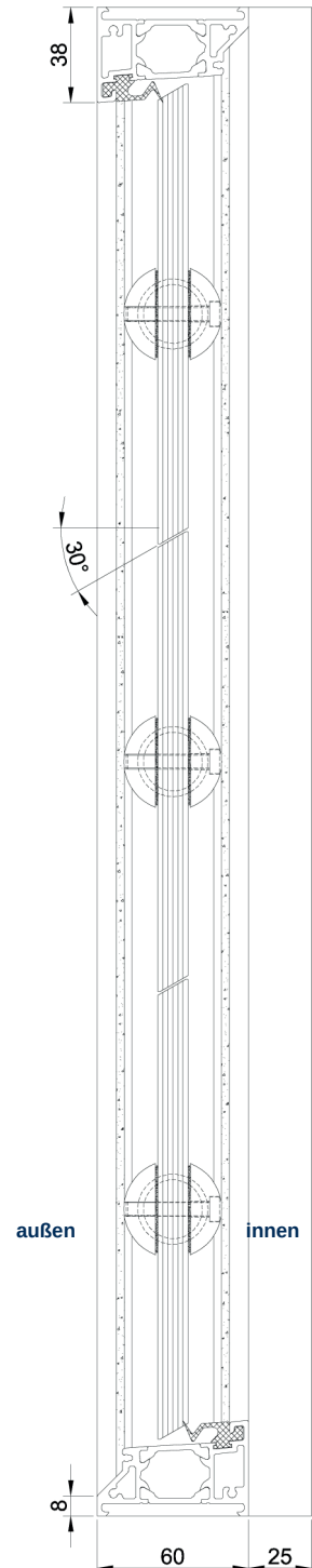
Vertikalschnitt (dargestellt ohne Bedienelement)
