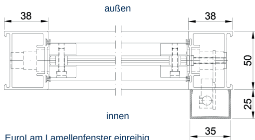
EuroLam Lamellenfenster einreihig
