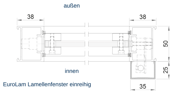
Horizontalschnitt einreihig (dargestellt ohne Bedienelement)
