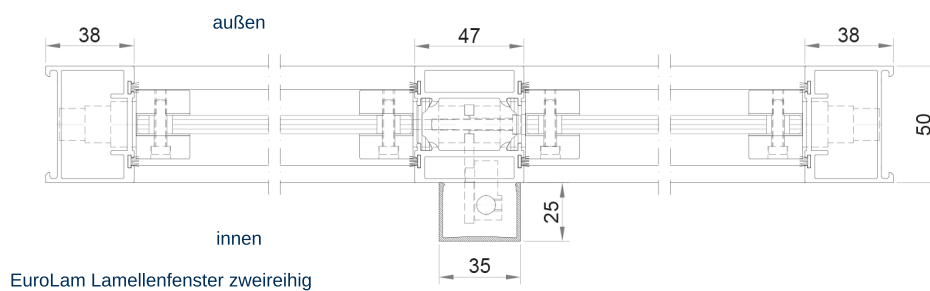
Horizontalschnitt zweireihig (dargestellt ohne Bedienelement)
