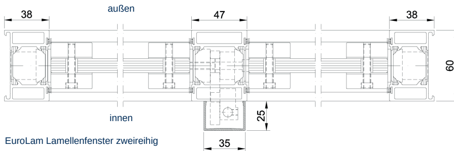
Horizontalschnitt zweireihig (dargestellt ohne Bedienelement)
