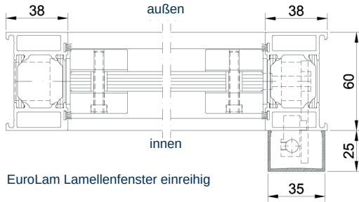
Horizontalschnitt einreihig (dargestellt ohne Bedienelement)
